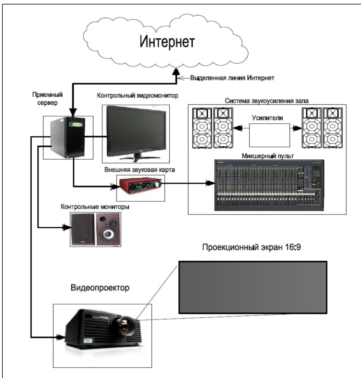
Рис. 1. Типовой технический комплекс ВКЗ
